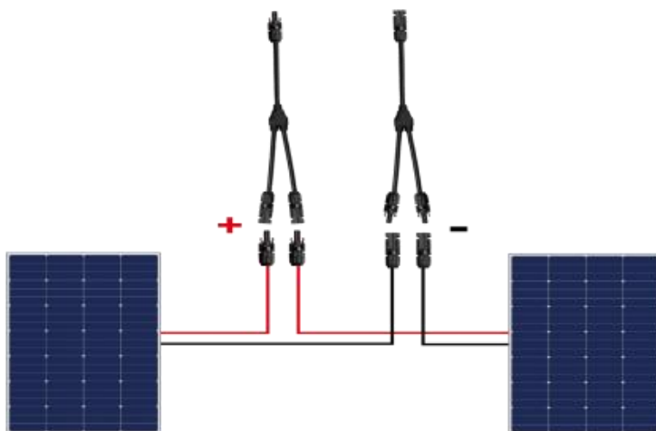
Schema di collegamento in parallelo di 400W*2:
