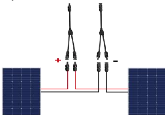
Schema di collegamento in parallelo 100W*2:
