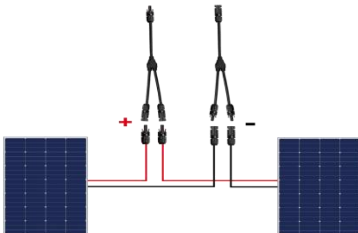
Schemat połączenia równoległego 400W*2:
