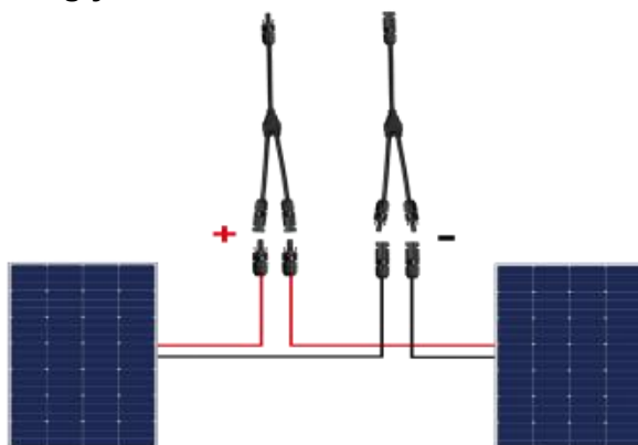
Schemat równoległy 100W*2:
