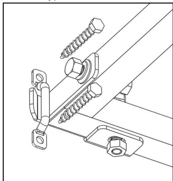
Śruba blokująca.
