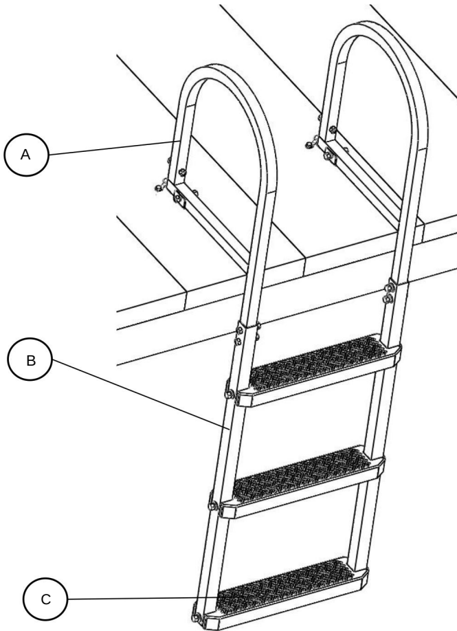
A: Handlauf B: Rahmen C: Stufe
