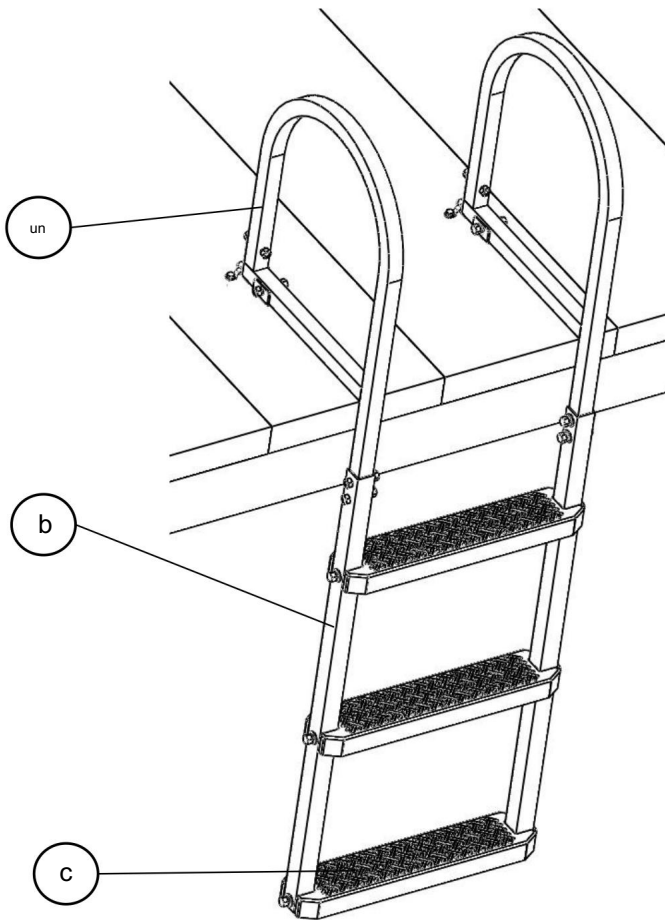
A : Rambarde B : Cadre C : Marche
