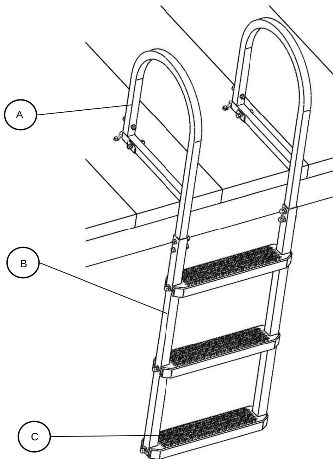
A: Leuning B: Frame C: Trede
